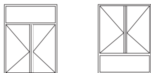
Française 2 vantaux avec imposte
